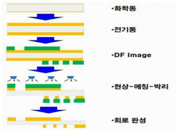
[그림 105] Tenting 공법: 에칭으로 회로 형성
