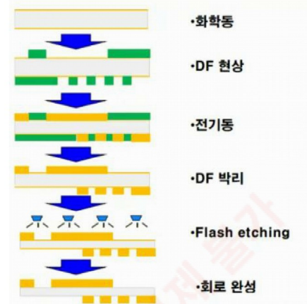
[그림 106] MSAP 공법: 노광, 현상으로 회로 형성
